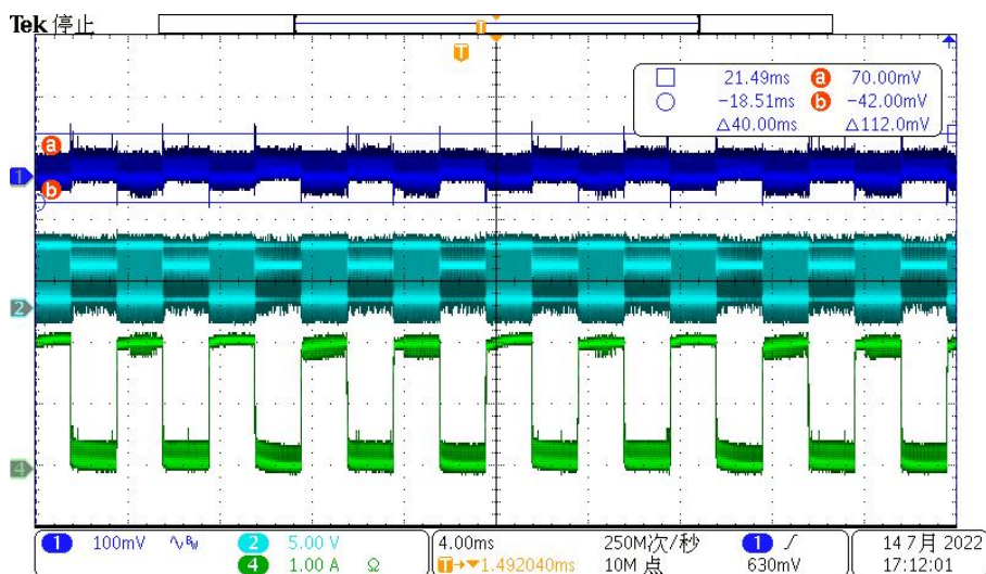
负载瞬态响应
