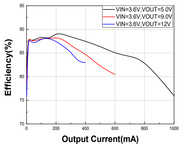
效率曲线
